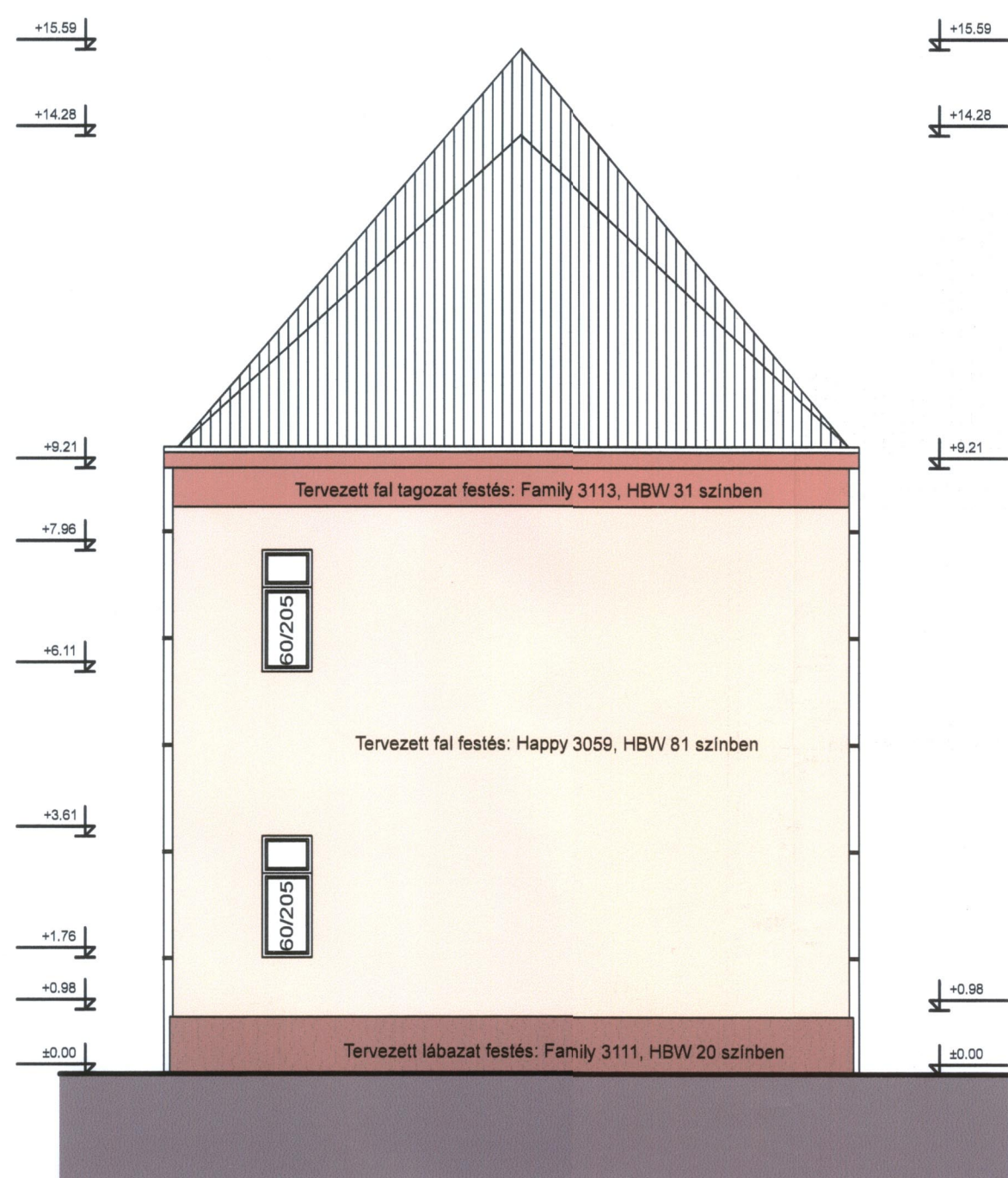
Kapubejáró felőli oldalsó homlokzat (Iskola) M=1:100
