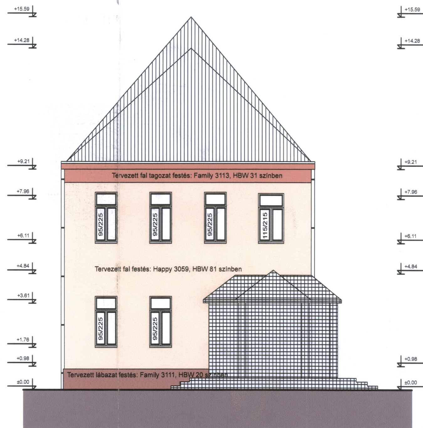
Iskola oldalsó homlokzat (Petőfi S. u. mellett) M=1:100
