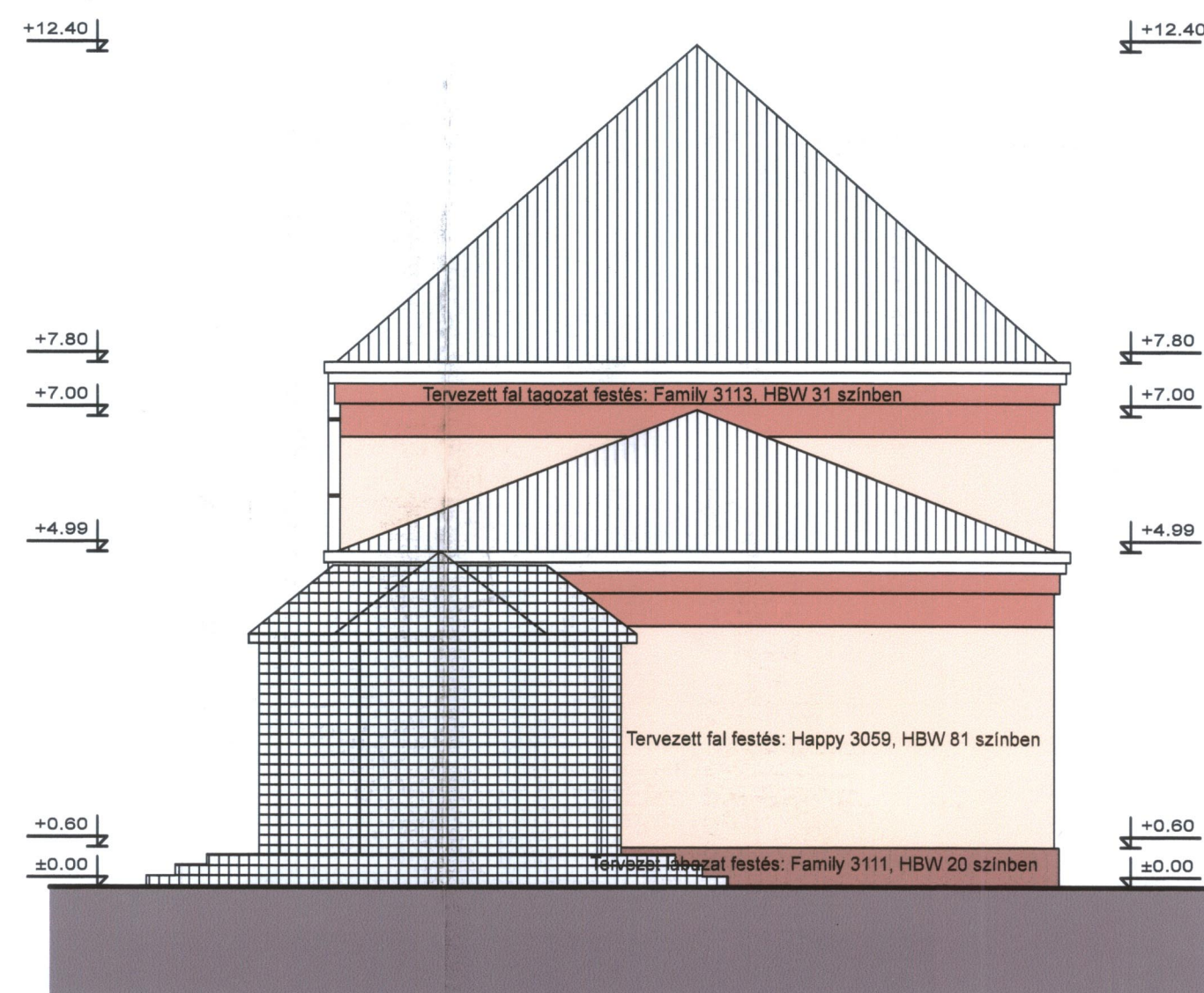
Tornaterem oldalsó homlokzat (Petőfi S. u. mellett) M=1:100
