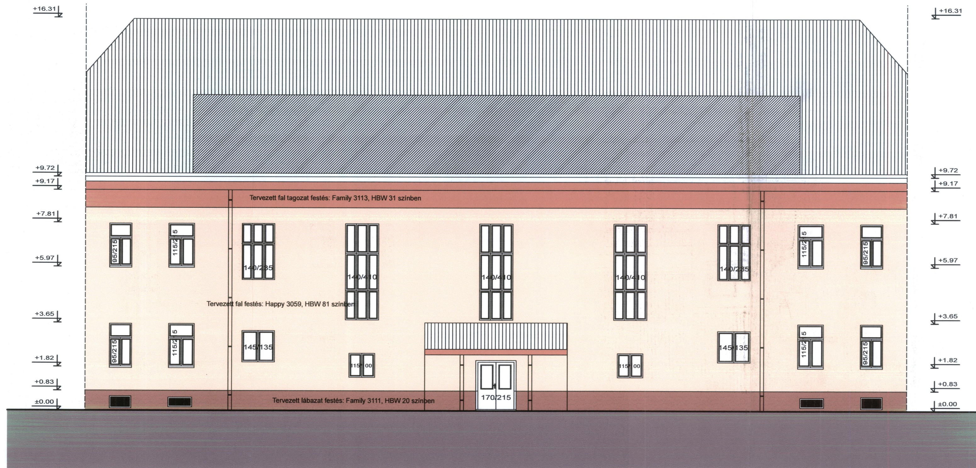
Kifordított belső íves homlokzat M=1:100
