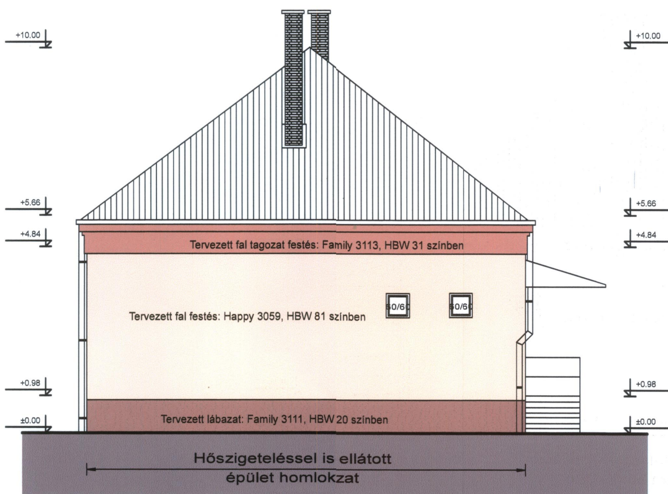
Kapubejáró felőli oldalsó homlokzat (tálaló konyha és ebédlő) M=1:100
